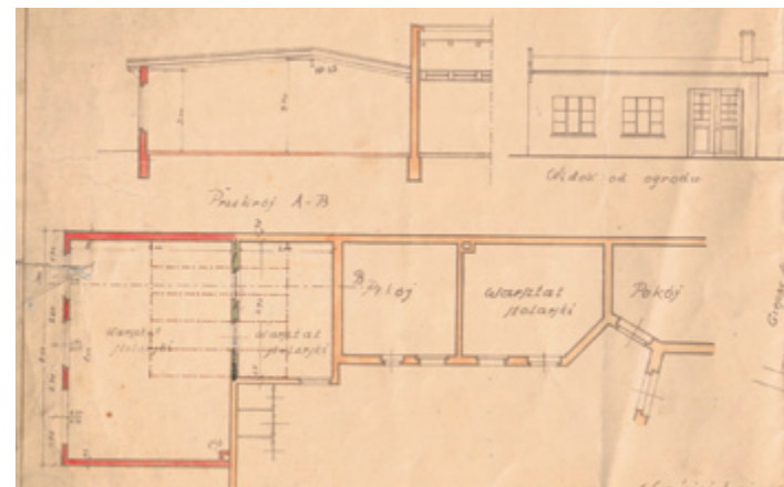
Fragment projektu rozbudowy warsztatu stolarskiego, 1938 r.; ze zbiorów Elżbiety Olejnik
